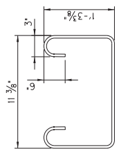
#6S3(E) BAR
